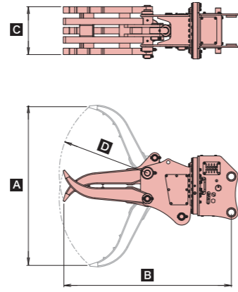
■全旋回グラスパー ダイナ 仕様図
