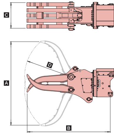
■完全油圧式ワンキャッチ専用 全旋回グラスパーVS 仕様図
