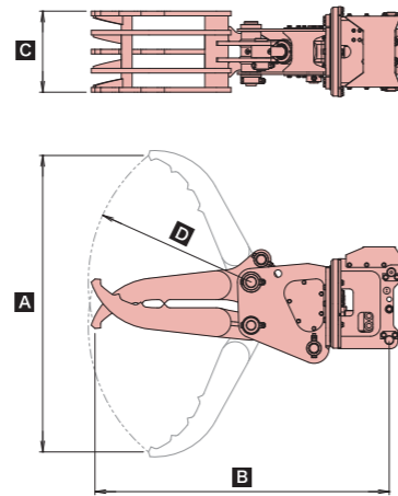
■完全油圧式ワンキャッチ プラス専用 全旋回グラスパー 仕様図
