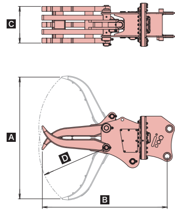
■全旋回グラスパー ソル 仕様図
