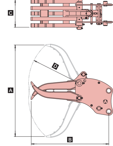
■首振りグラスパーVL 仕様図
