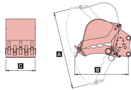
■CBRB-L(バケット仕様) 仕様図
